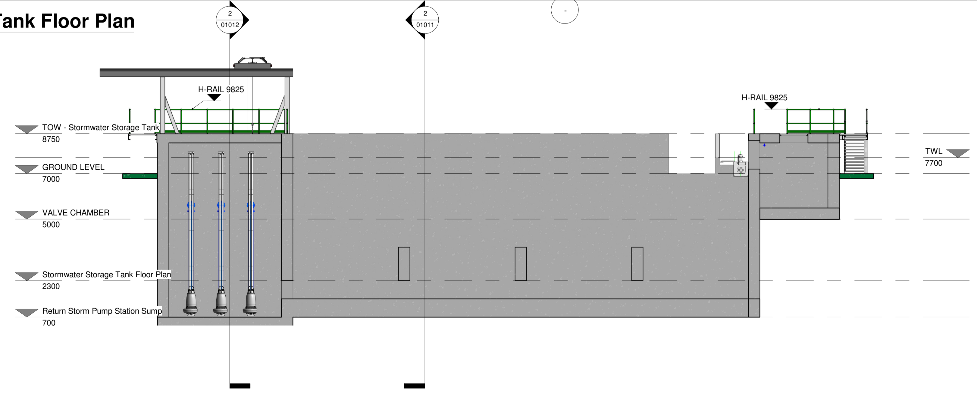
2 Section 1 1 : 100
